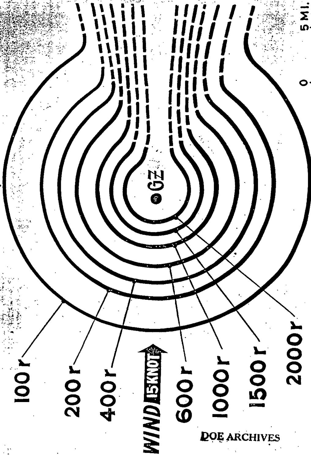
FIG.5 GZ CONTOURS 15 MT (LAND)
